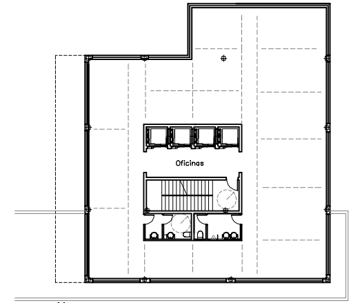
Planta 3 -oficinas-
