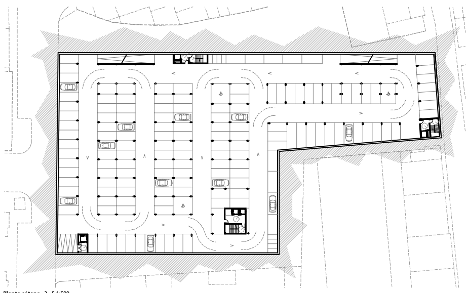
Planta sótano -2 E.1/500
