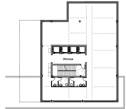
Planta 2 -oficinas-
