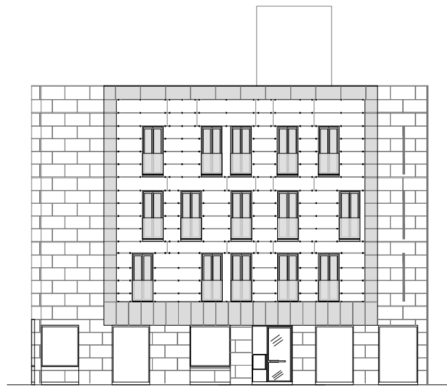
AIZADO PRINCIPAL
