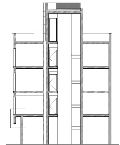
SECCIÓN A-A'
