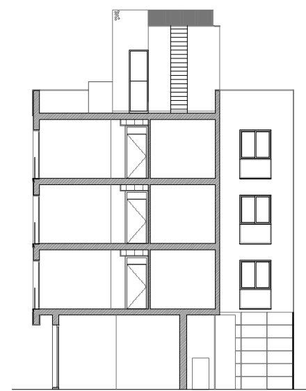
SECCIÓN C-C'
